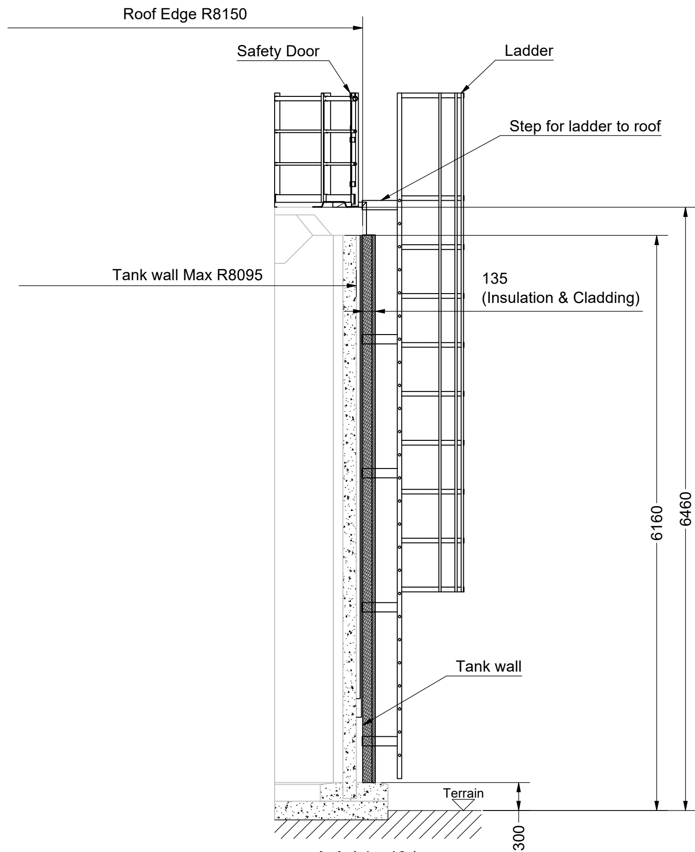
B-B ( 1 : 12,5 )
